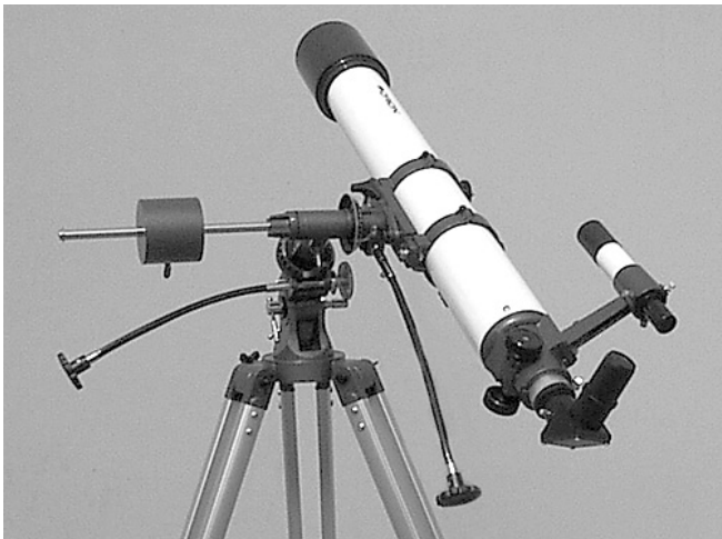
Figure 5a. Télescope orienté vers le sud. Notez que sur toutes ces illustrations, la monture et le trépied restent immobiles. Seuls les axes d'ascension droite et de déclinaison se déplacent.
