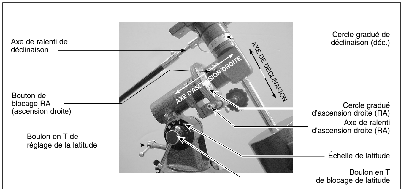
Figure 2. La monture équatoriale
