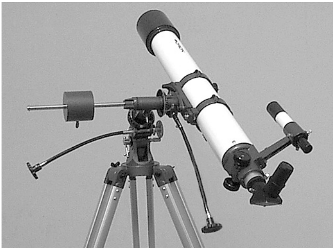
Figura 5a. Telescopio apuntando al sur. Tenga en cuenta que en todos estos ejemplos, la montura y el trípode permanecen estacionarios, solo los ejes de A. R. y Dec. se mueven.
