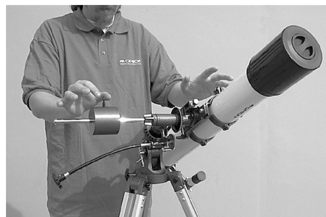
Figura 3b. Ahora el telescopio estará equilibrado respecto al eje de ascensión recta. Es decir, al soltar las manos, el eje de contrapeso se mantiene en posición horizontal.
